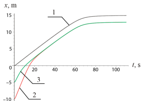
Рис. 3. Изменение проекции вектора перемещения группы роботов на ось X
