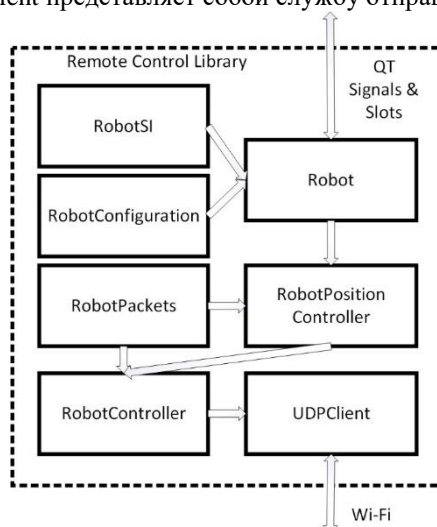
Рис. 3. Схема библиотеки внешнего управления
