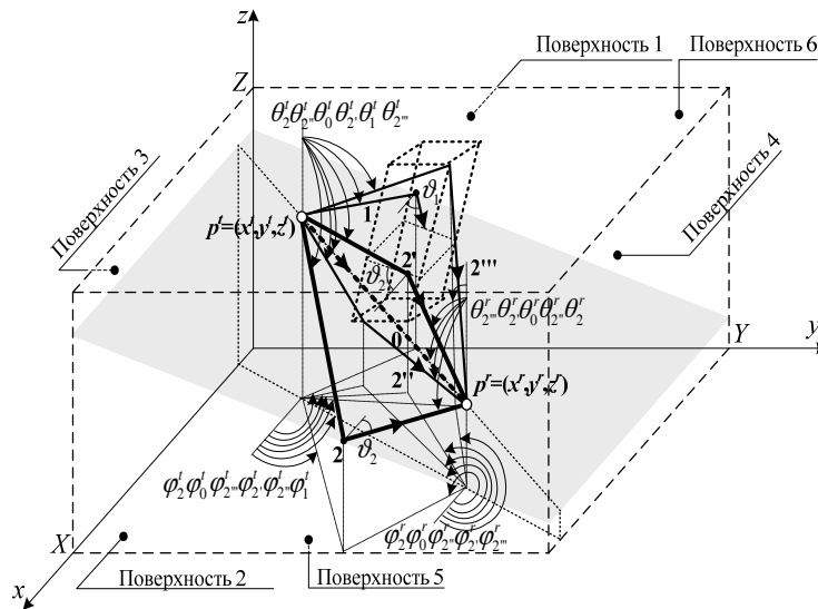
Рис. 3. Основные геометрические параметры кластера
