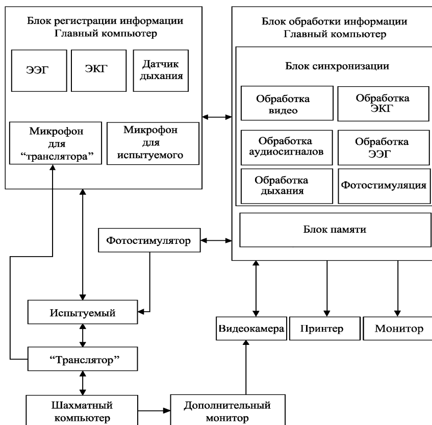
Рис. 1. Структура биотехнической системы
